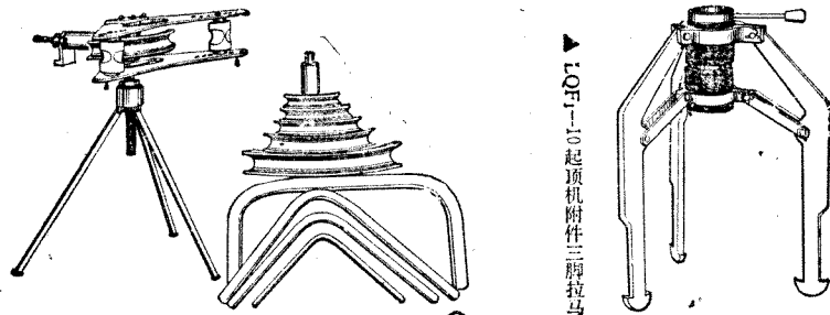
▲ LWG1-10B 分离式三脚架液压弯管机
