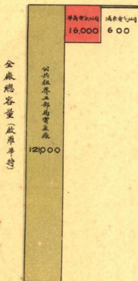
總容量及每度所需煤量比較圖
