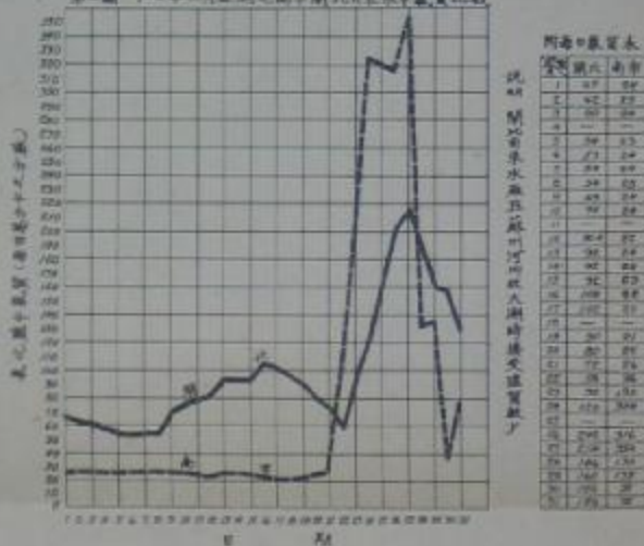
第二圖 十七年二月間潮之南閘北自來水中氣質比較
