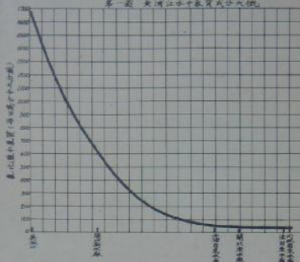
第一圖 黃浦江水中氣質成分大體
